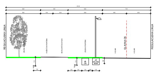
PRESJEK 5-5
