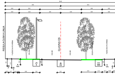
PRESJEK 9 - 9
