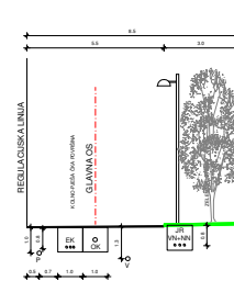
PRESJEK 10-10
