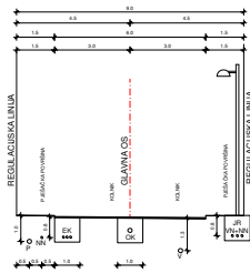
PRESJEK 4-4
