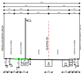
PRESJEK 3-3
