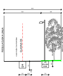
PRESJEK 6-6
