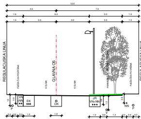
PRESJEK 2-2
