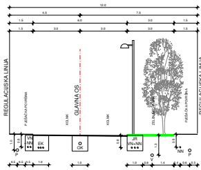
PRESJEK 1-1
