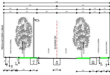
PRESJEK 8 - 8
