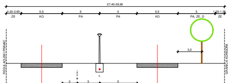
PRESJEK J
