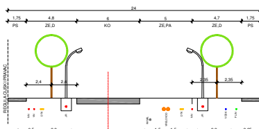
PRESJEK E
