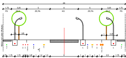
PRESJEK D
