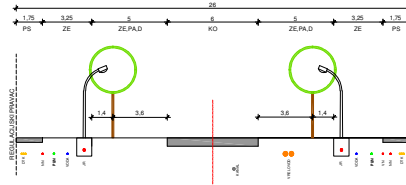
PRESJEK F
