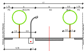
PRESJEK G
