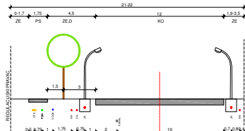
PRESJEK A
