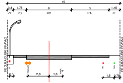
PRESJEK I
