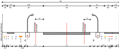
PRESJEK H
