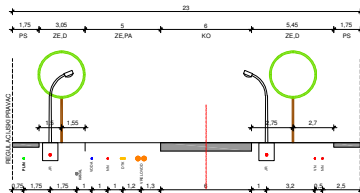
PRESJEK B
