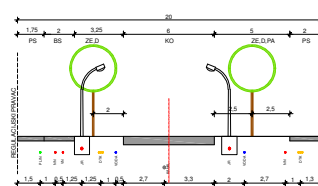
PRESJEK F
